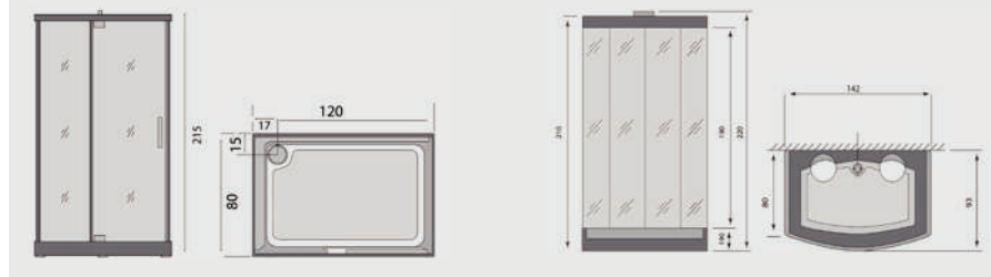
کابین سونای بنیتا R۹۸۵ - L۹۸۶ (چپ و راست) Benita L986 - R985 ابعاد: ۲۱۵ × ۸۰ × ۱۲۰ سانتیمتر سونا بخار، ماساژور بدن صفحه کنترل دیجیتال، کنترل دما و زمان سونای بخار، سیستم محافظ جان، تلفن، رادیو پمپ تامین فشار آب، ضد عفونی کننده آزن، تهویه دوش دستی، دوش سقفی، آینه، روشنایی شیشه نانو برق مصرفی سونا ۳۰۰۰ وات
