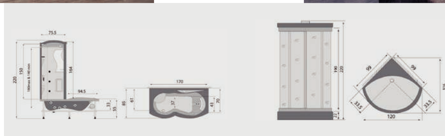
نیم کابین هلنا ۲۵۹ (چپ و راست) ابعاد: ۲۲۰ × ۷۰ (۸۵) × ۱۷۰ سانتیمتر جکوزی، ماساژور بدن، ماساژور پا صفحه کنترل دیجیتال، سیستم محافظ جان دوش دستی، دوش سقفی، آینه، روشنایی، تهویه برق مصرفی جکوزی ۱۱۰۰ وات
