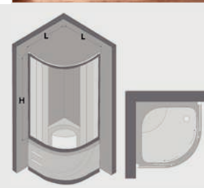
مینی وان لاریسا و دور دوشی ۱۳۰ ابعاد: ۹۱ × ۹۱ × ۴۹ (۳۰۱) سانتیمتر شیشه: شفاف / مات دوردوشی: فریم سفید Larisa 130
